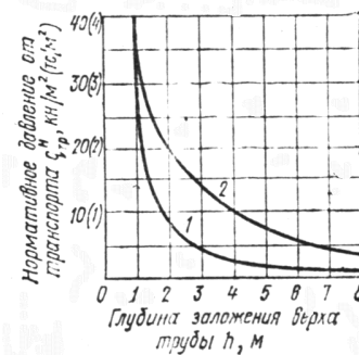
Рис. 1 Зависимость нормативного равномерно распределенного давления транспорта q^H_{Тр} от глубины заложения трубопровода
